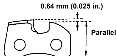
(Depth gauge)
