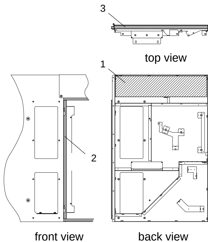
Rear bonnet : left
