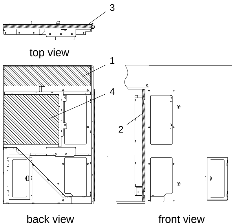
Rear bonnet : right
