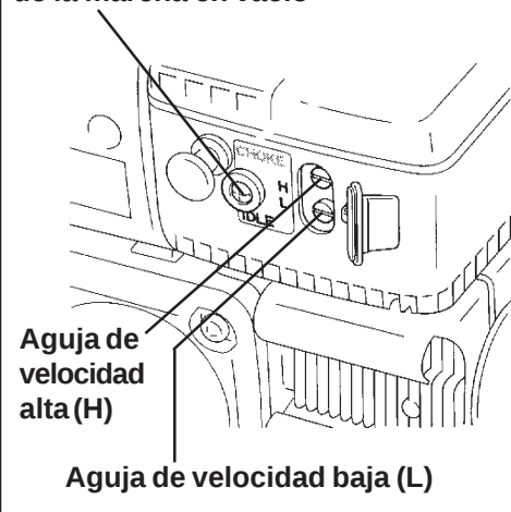
Tornillo de ajuste de la velocidad de la marcha en vacío
